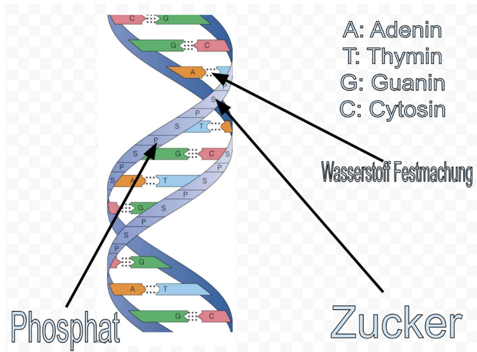
Diagramm von DNA (oben)
