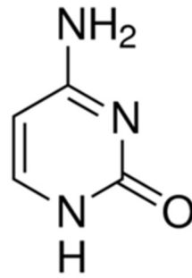
Cytosin
