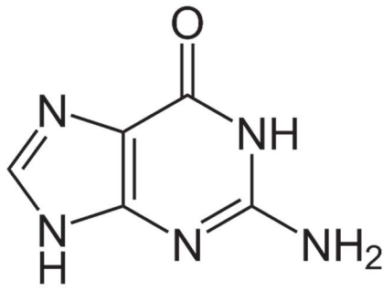
Guanin
