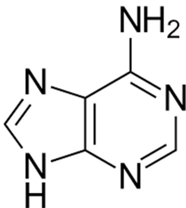
Adenin
